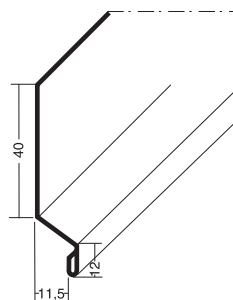
Waterslagprofiel
